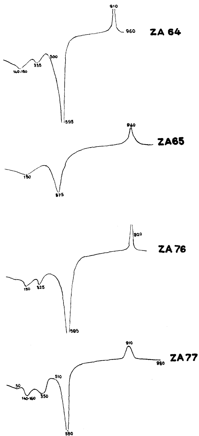
Fig. 6 - Courbes d'analyse thermique différentielle (Argiles ZOMANDAO)
