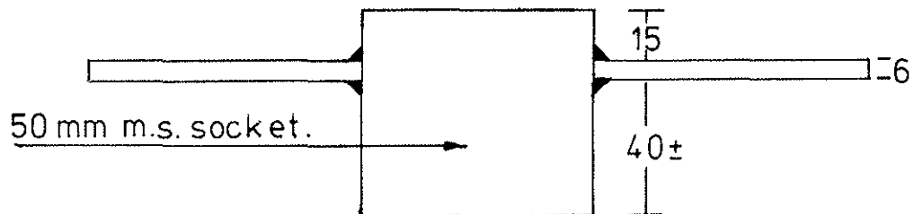
hanger plate - section AA.
